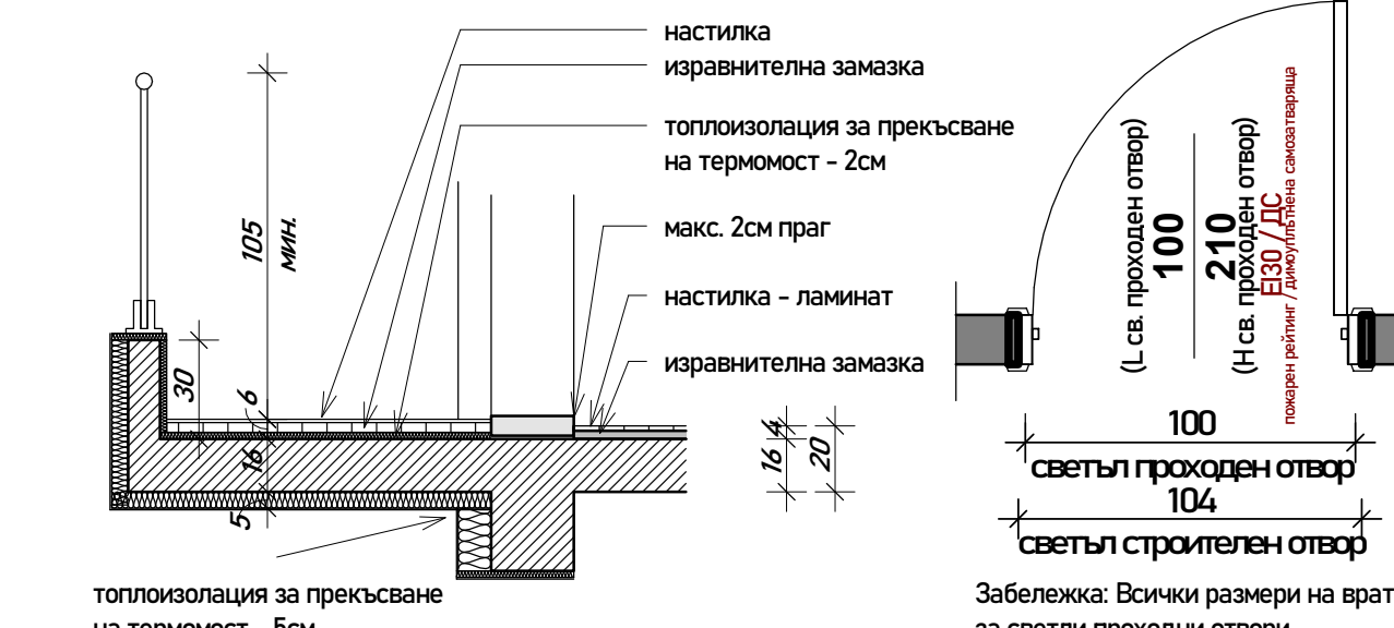
детайл балкони 1:25 интериорни врати 1:25
