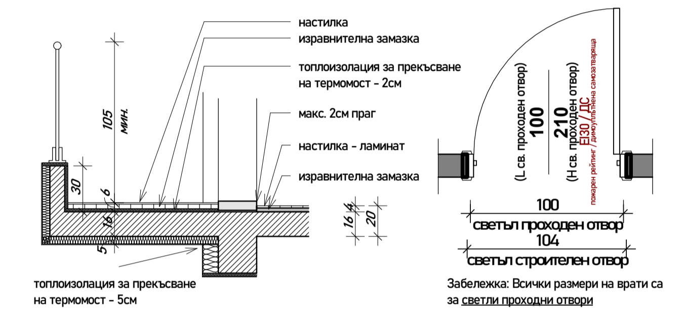
детайл балкони 1:25 интериорни врати 1:25
